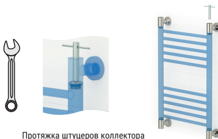
Протяжка штуцеров коллектора
