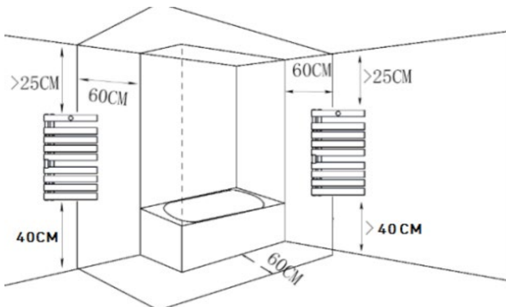
Рисунок 2. Монтажные отступы
