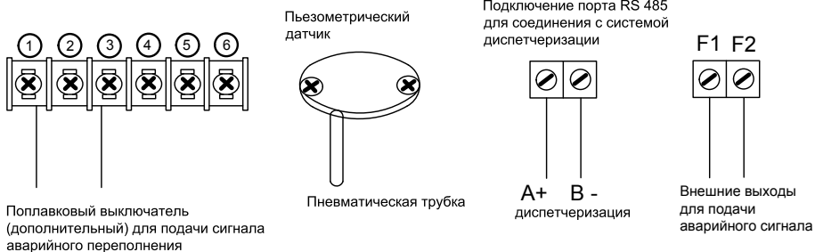
Рис. 13 Подключение реле уровня, порта диспетчеризации, внешней аварийной сигнализации
